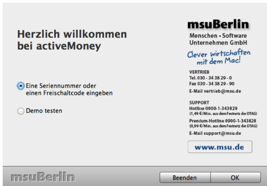
Arbeitsmodus auswählen
