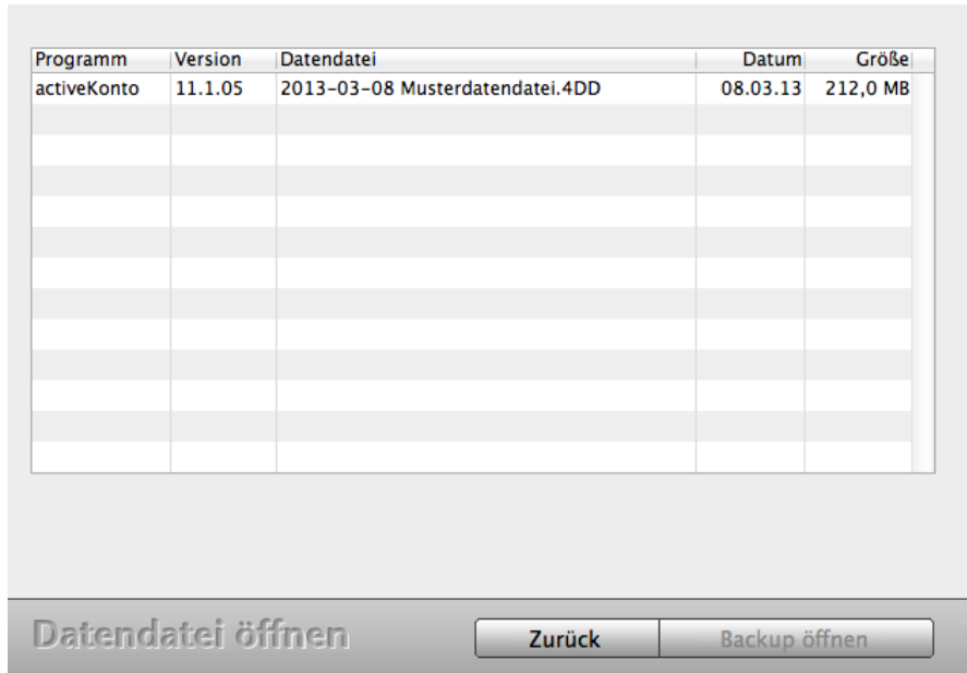
Backup öffnen-Auswahldialog
