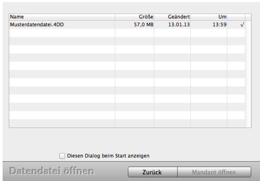
Mandant wechseln-Auswahldialog
