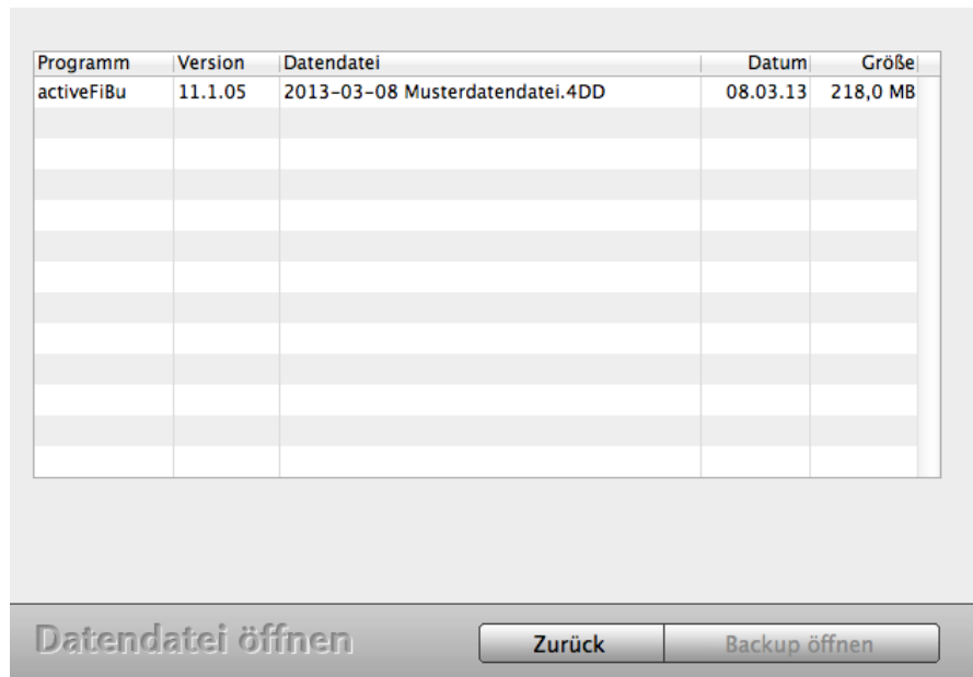
Backup öffnen-Auswahldialog
