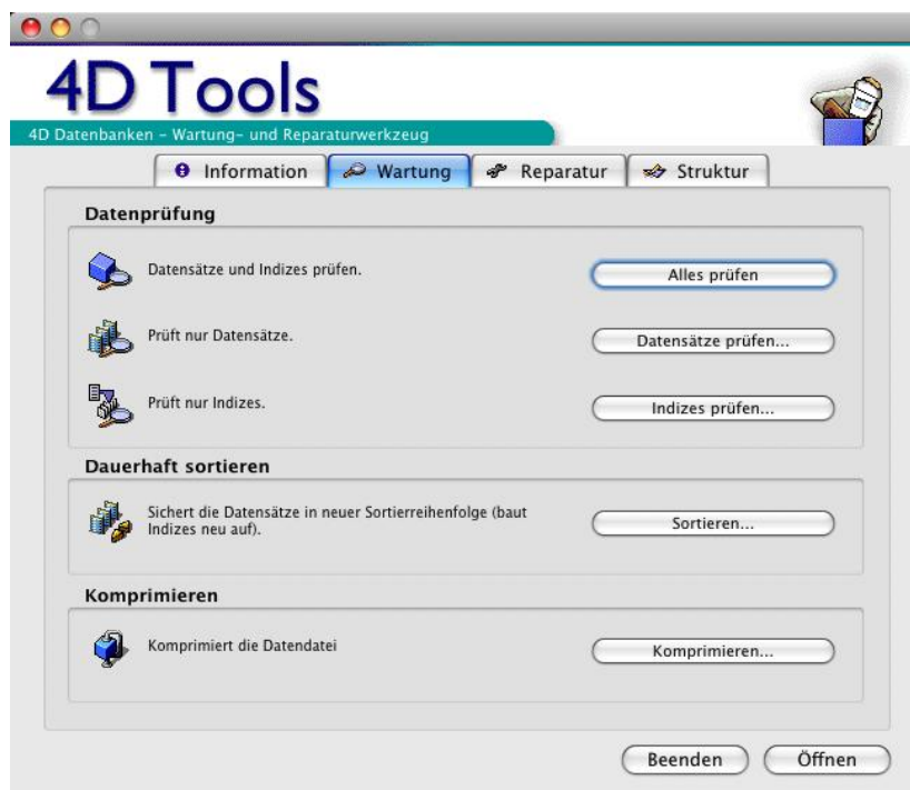
msuWartung - Komprimieren
