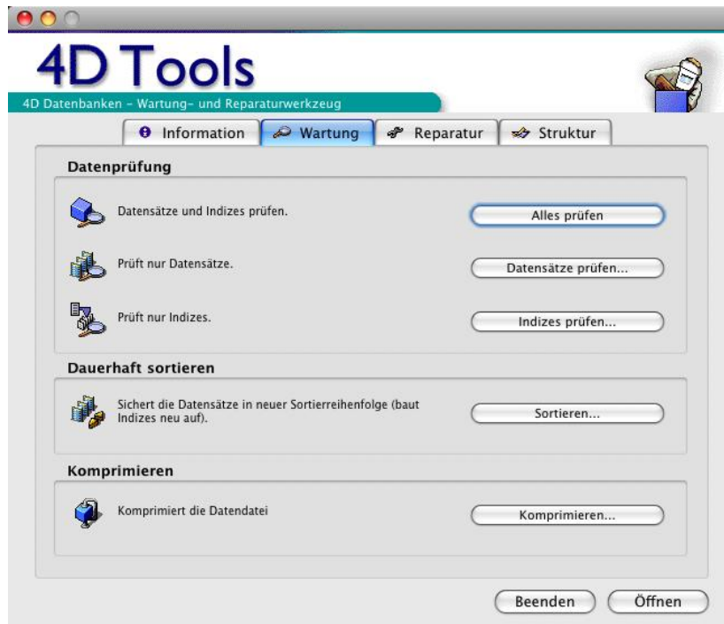
msuWartung - Komprimieren
